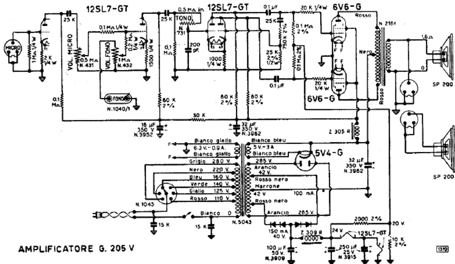
Lo schema elettrico.
